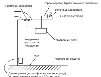
Рис. 4. Магистраль хладагента перекрывается по сигналу датчика хладагента
