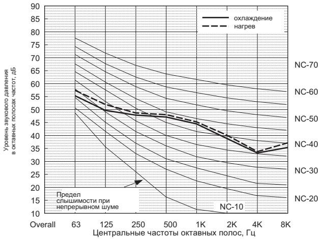
Уровень шума PUMY-P100YHMB, VHMB
