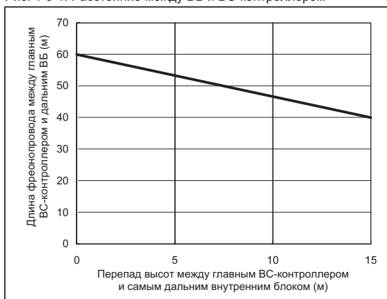
Рис. 4-3-1. Расстояние между ВБ и ВС-контроллером
