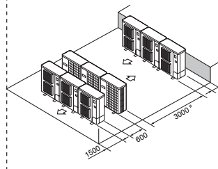
Рис. 12. Установка рядами. * Если установлена решетка, изменяющая направление выброса воздуха, то расстояние можно уменьшить до 1500 мм.
