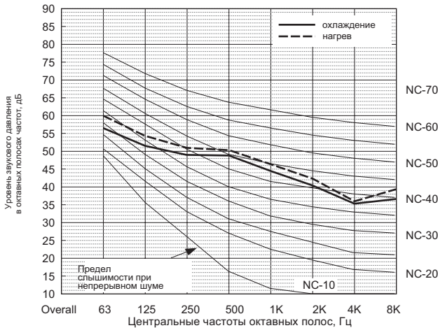
Уровень шума PUMY-P125YHMB, VHMB
