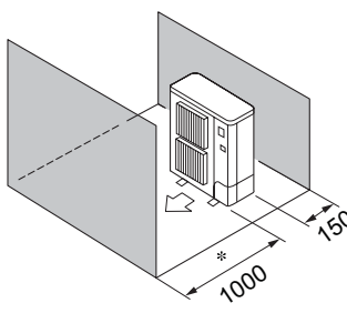
Рис. 6. Препятствие сзади и спереди. * Если установлена решетка, изменяющая направление выброса воздуха, то расстояние можно уменьшить до 500 мм.
